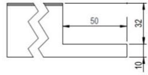
Verstärkungswinkel: 1x wie gezeichnet, 1x gegengleich
