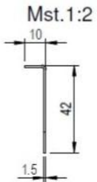
Verstärkungswinkel: 1x wie gezeichnet, 1x gegengleich
